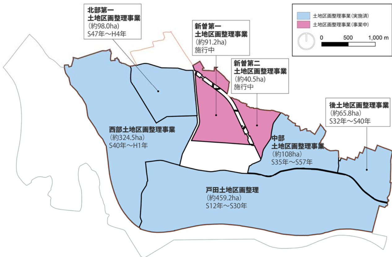
図 1-22 土地区画整理事業（施行中）の位置
