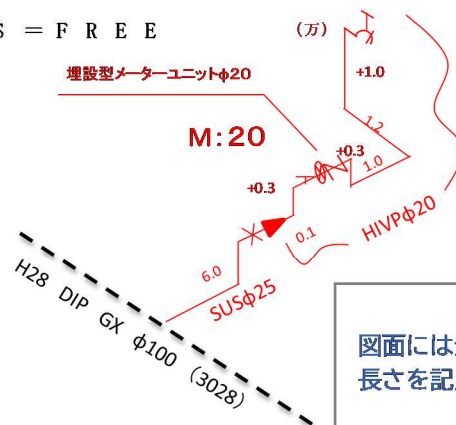
立面图
