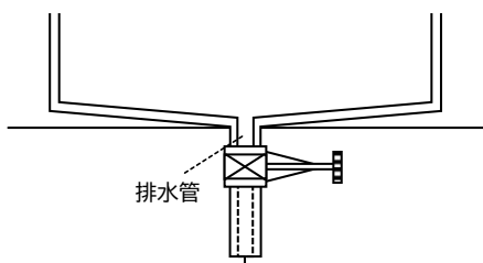
◇ 参考事項図-1.10 蓄圧式給水タンク
