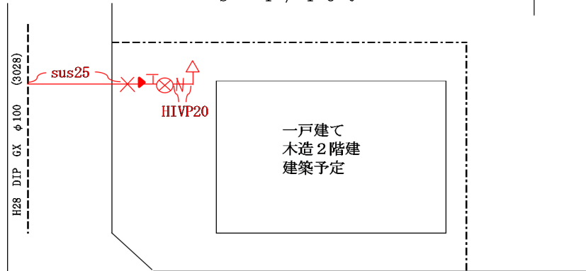
平面图
