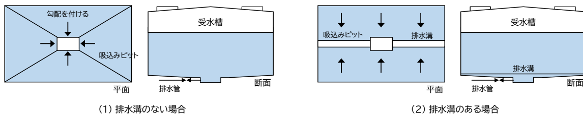
◇ 参考事項図-1.5 排水管取付けの一例（給排水設備基準・解説 2006 年版（財）日本建築センター）
