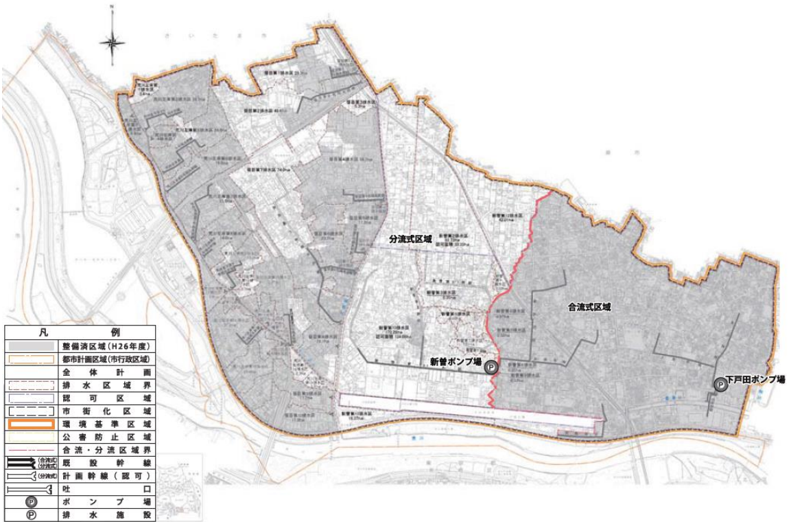
図 2－113 公共下水道事業計画図（雨水）
